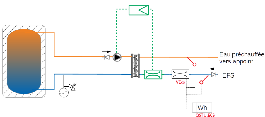
Figure 3 : Régulation par un dispositif de détection ou de mesure de débit
